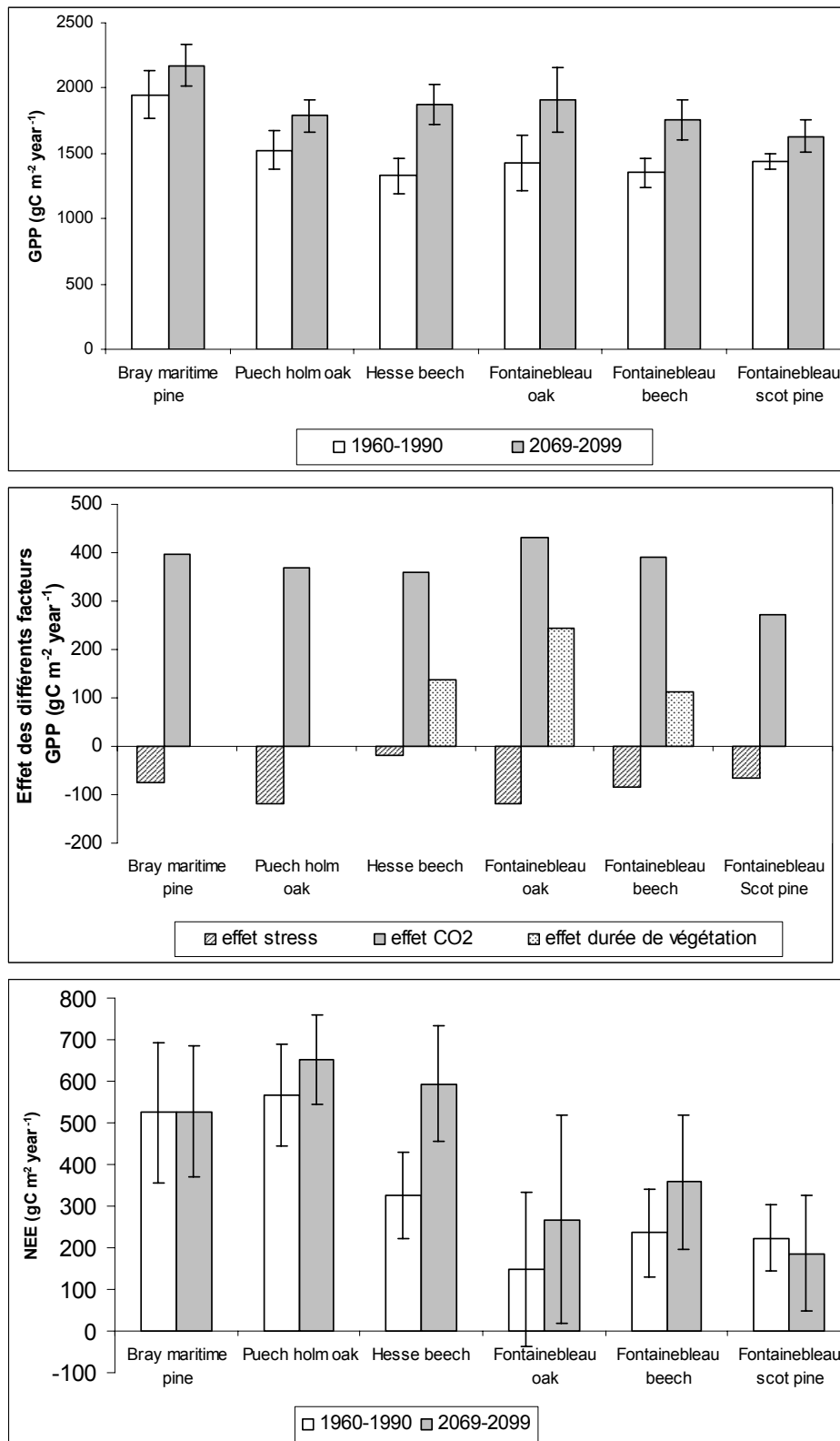
Figure 9bis: comparaison des moyennes simulées annuelles entre 1960-1990 et 2069-2099 sur les 6 peuplements étudiés. En haut la production primaire brute (GPP), au centre les effets du changement climatique sur la GPP, en bas le flux net de CO 2 (NEE).
