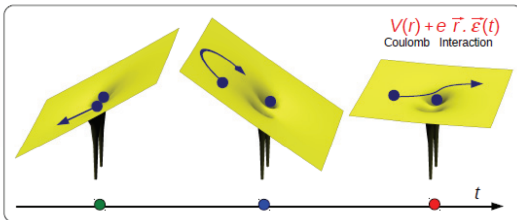
P.B. Corkum PRL 71, 1994 (1993)
